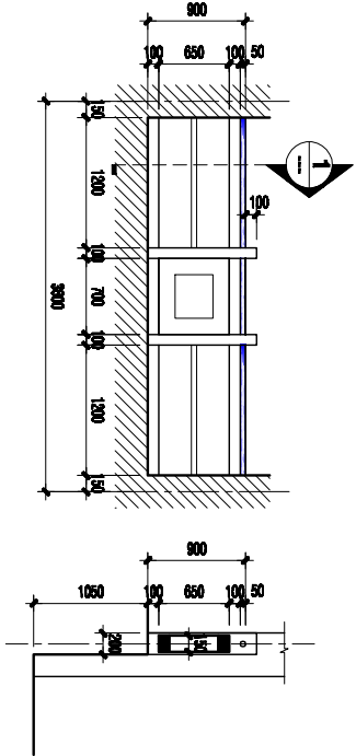
LAN CAN ĐIỆN HÌNH TL: 1/50
