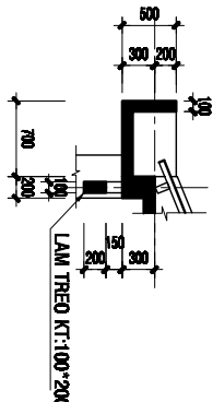
SẾ NỒ, LAM TREO TL: 1/50
