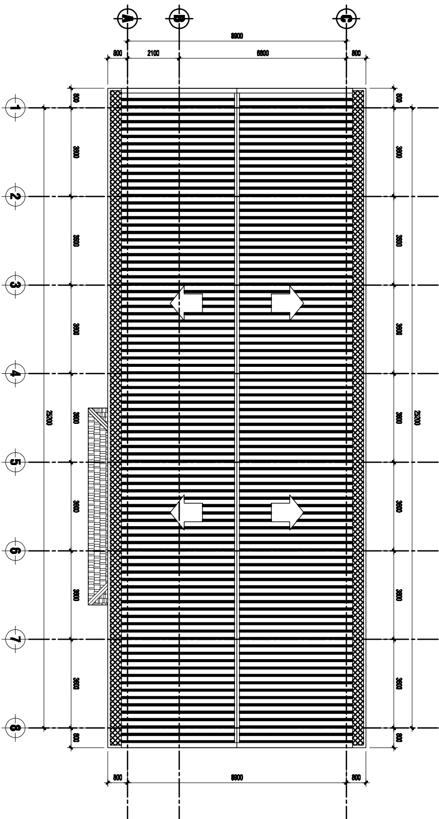
MẶT BẰNG MÁI HIỆN TRẠNG TL: 1/100
