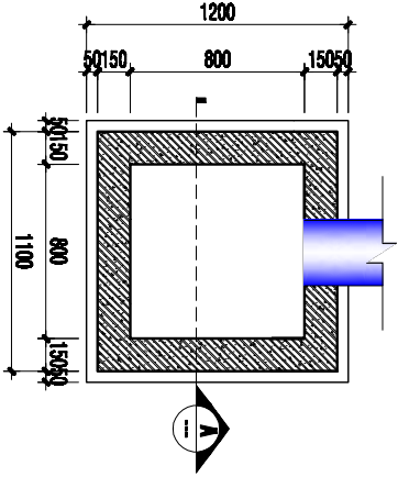
THIỆP HỒ GA TL: 1/25 (SL: 02CK)
