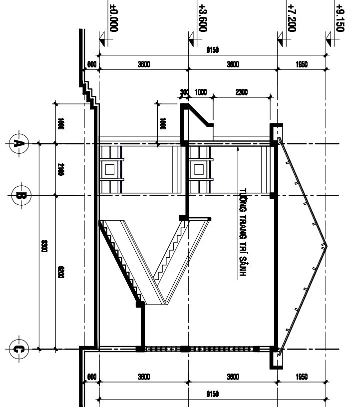
MẶT CẮT A-A HIỆN TRẠNG TL: 1/100
