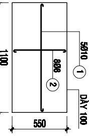
THIỆP HỒ GA TL: 1/25 (SL: 02CK)
