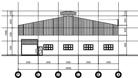
MẶT ĐỨNG TRỤC F-A KHO HÀNG 3 TỶ LỆ 1/100
