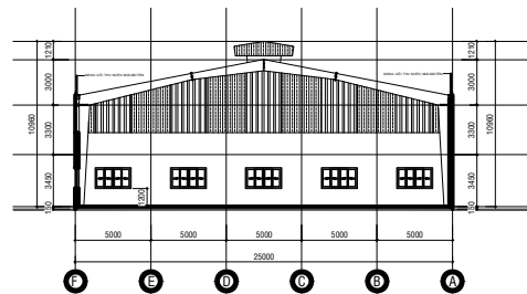
MẶT CẮT B-B
