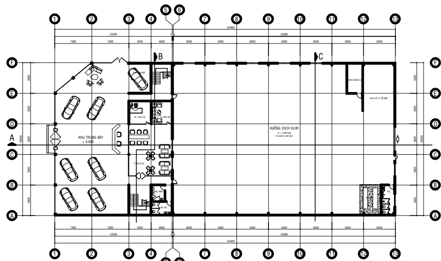
MẶT BẰNG TẦNG 1 SHOWROOM A1 + XƯỞNG DỊCH VỤ B1 TỶ LỆ 1/100
