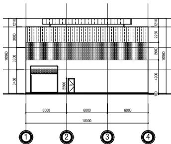
MẶT ĐỨNG TRỤC 1-5 KHO HÀNG 3 TỶ LỆ 1/100
