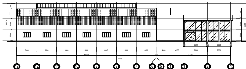
MẶT ĐỨNG TRỰC 13-1 SHOWROOM A1 + XƯỞNG DỊCH VỤ B1 TỶ LỆ 1/100
