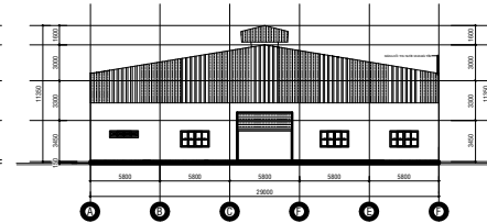
MẶT ĐỨNG TRỰC A-F TỶ LỆ 1/100
