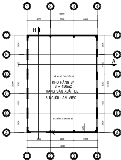
MẶT BẰNG KHO HÀNG 4 TỶ LỆ 1/100
