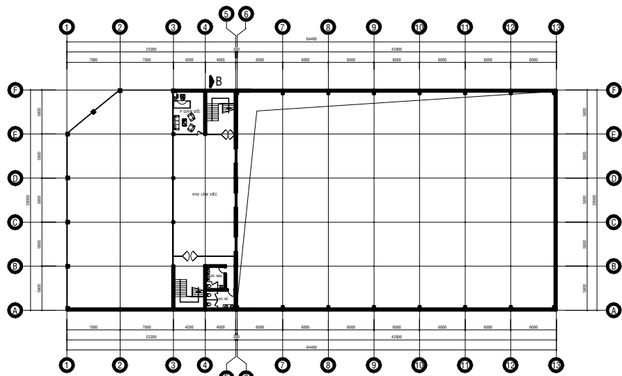
MẶT BẰNG TẦNG 2 SHOWROOM A1 + XƯỞNG DỊCH VỤ B1 TỶ LỆ 1/100
