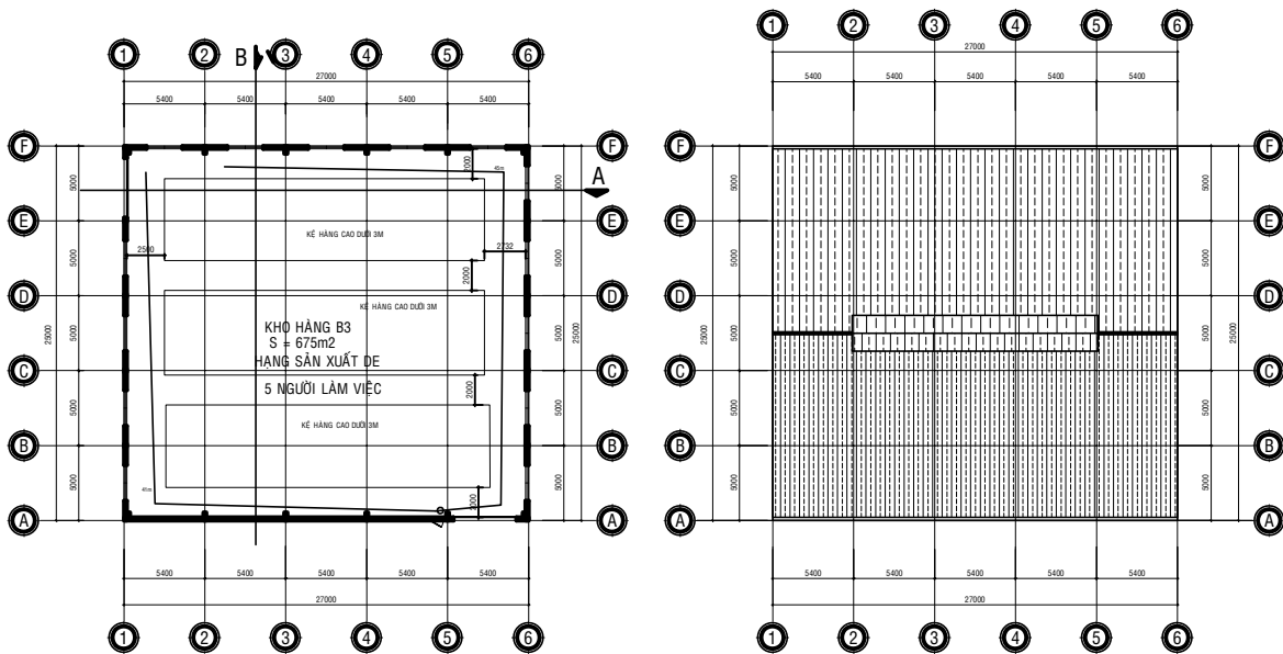
MẶT BẰNG KHO HÀNG 3 TỶ LỆ 1/100
