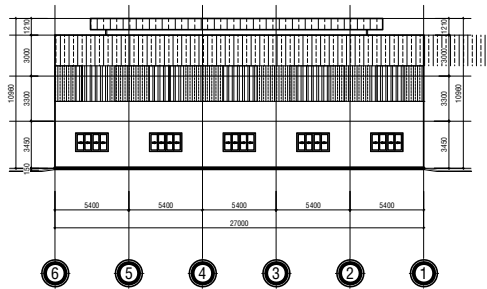
MẶT ĐỨNG TRỤC 6-1 KHO HÀNG 3 TỶ LỆ 1/100
