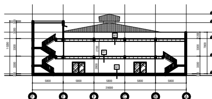
MẶT CẮT B-B
