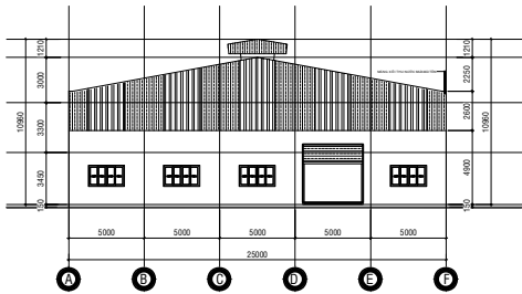
MẶT ĐỨNG TRỤC A-F KHO HÀNG 3 TỶ LỆ 1/100
