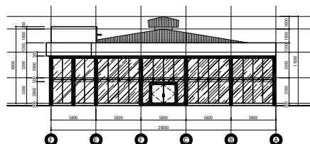
MẶT ĐỨNG TRỰC F-A TỶ LỆ 1/100
