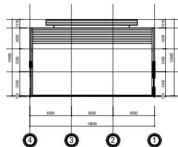
MẶT CẮT A-A
