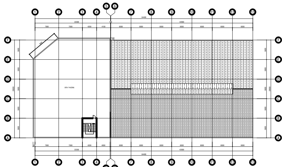
MẶT BẰNG TẦNG MÁI SHOWROOM A1 + XƯỞNG DỊCH VỤ B1 TỶ LỆ 1/100
