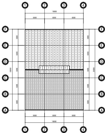
MẶT BẰNG KHO HÀNG 4 TỶ LỆ 1/100
