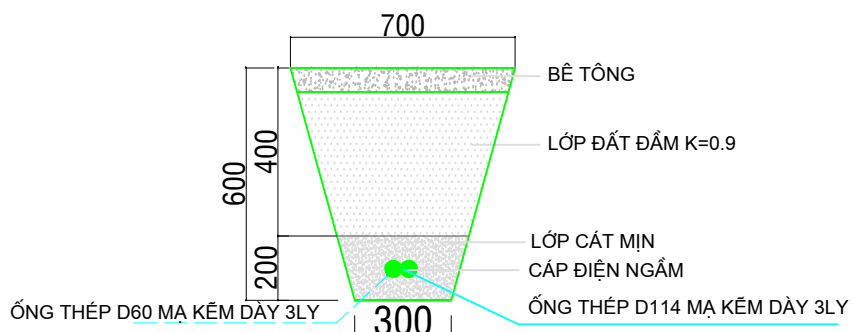
C.T MƯỜNG CHỖN CÁP ĐIỆN QUA ĐƯỜNG
