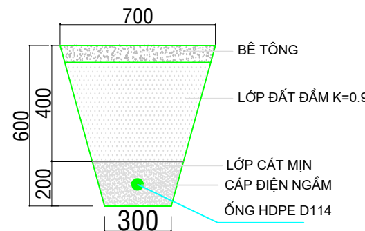
C.T MƯỜNG CHỖN CÁP ĐIỆN ĐI NGẦM (1 CẤP)
