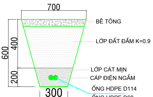
C.T MƯỜNG CHỖN CÁP ĐIỆN ĐI NGẦM (2 CẤP)
